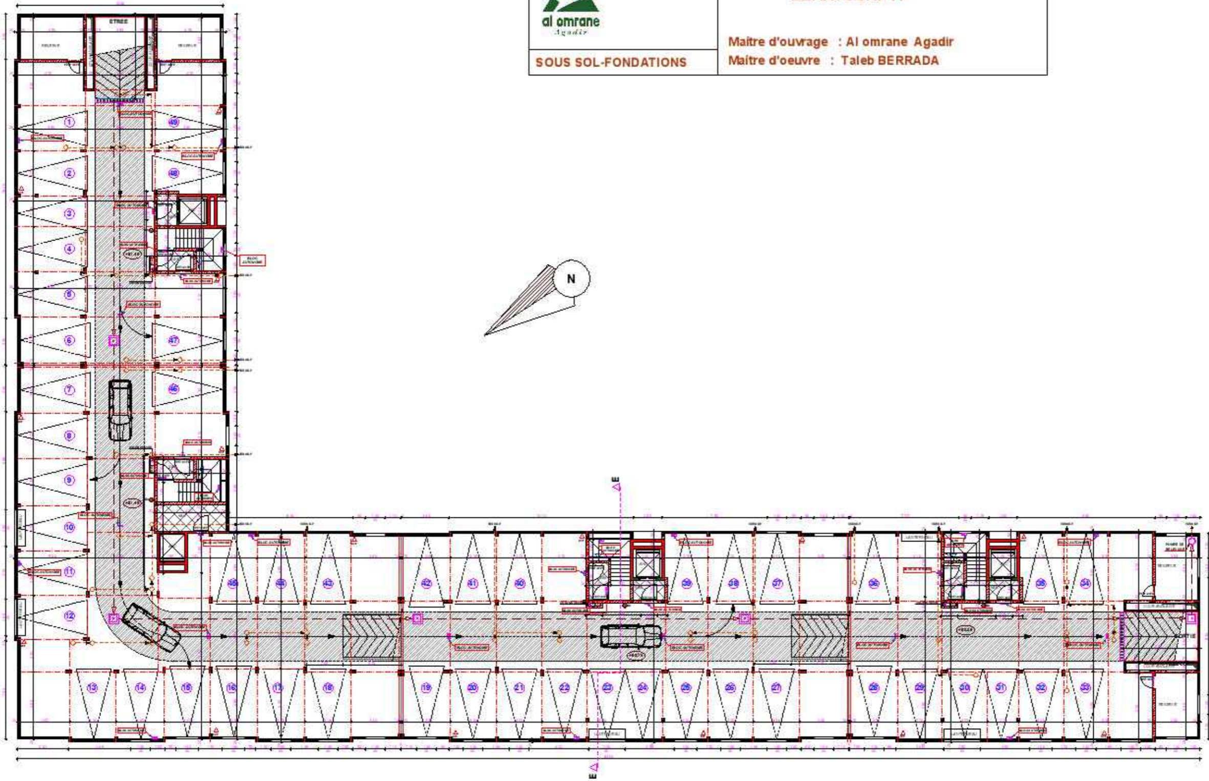
SOUS SOL - FONDATIONS
