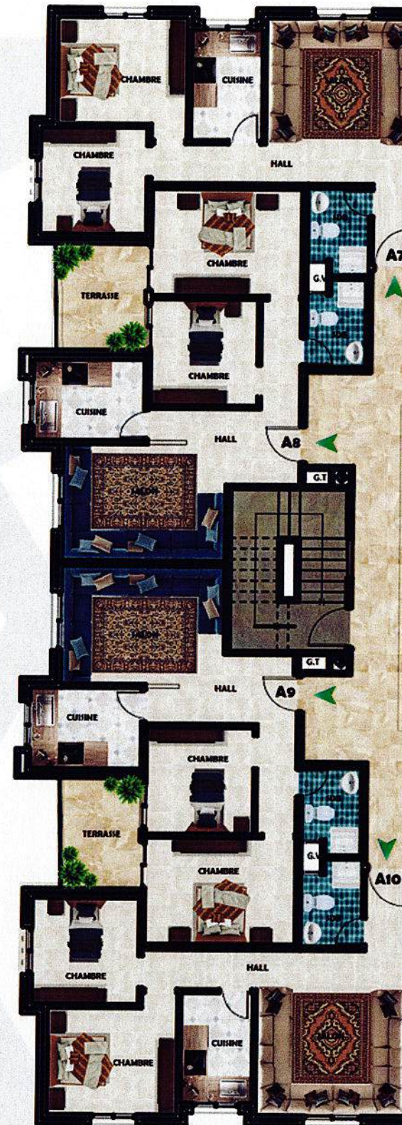
Plan 2ème ETAGE
