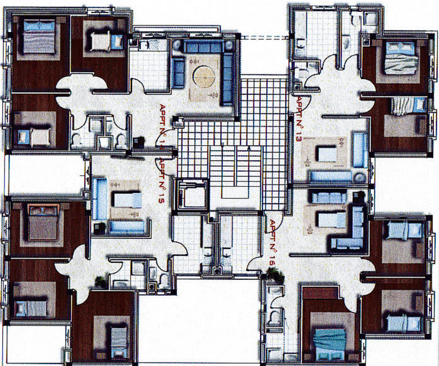
PLAN DU 3 ÈME ETAGE
