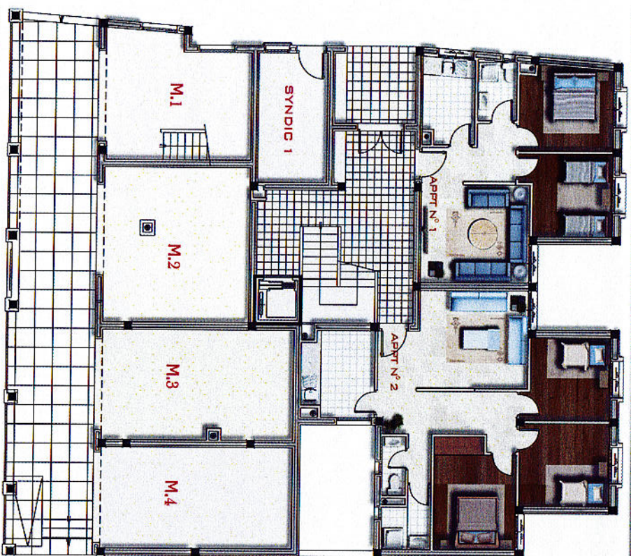
PLAN DU REZ-DE-CHAUSSEE
