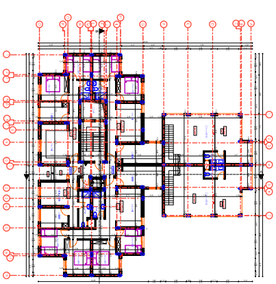
PLAN REZ DE CHAUSSEE
