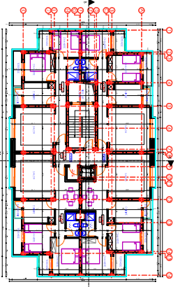
PLAN 1ER ETAGE
