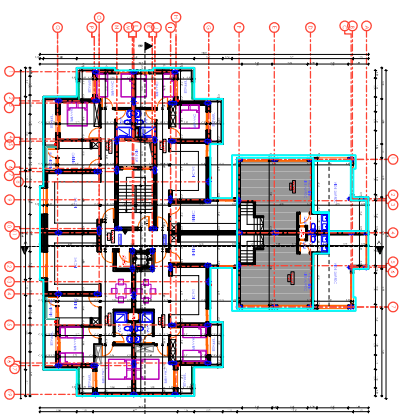
PLAN 1ER ETAGE
