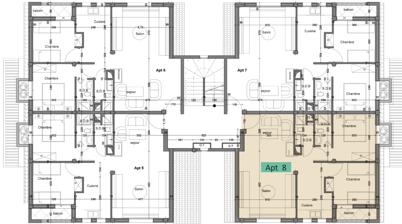
IMMEUBLE TYPE
