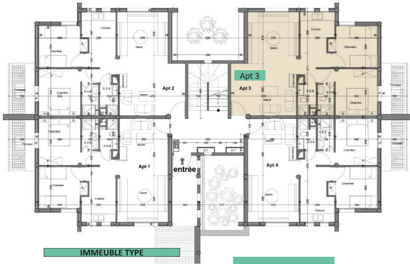
Plan RDC
