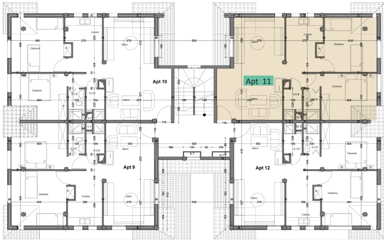
IMMEUBLE TYPE
