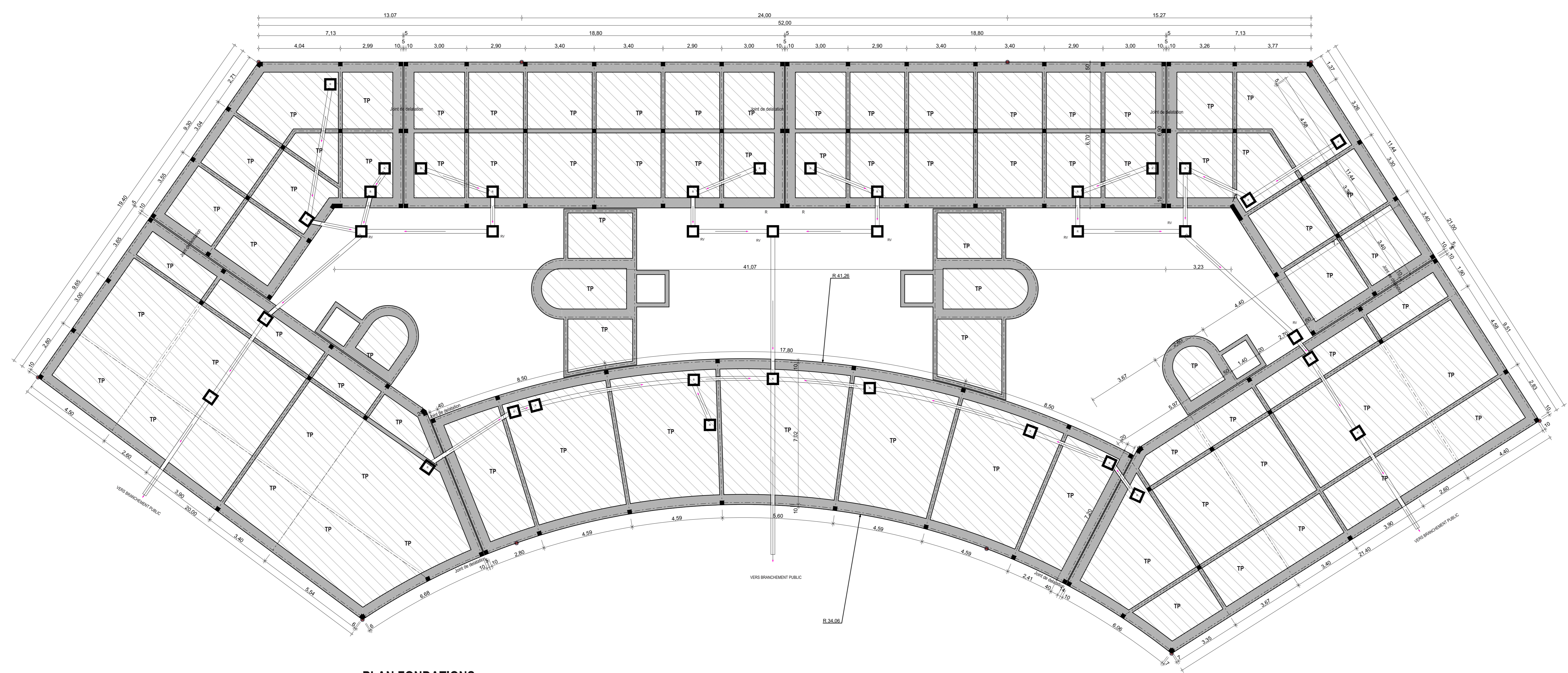
PLAN FONDATIONS
