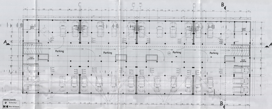
Sous sol Imm A/A'
