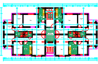
ETAGE COURANT
