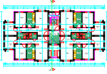
REZ DE CHAUSSEE
