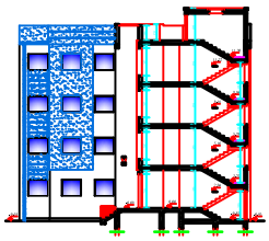
COUPE AA
