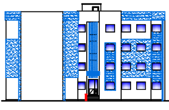
FACADE SUR ENTREE
