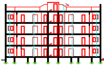
COUPE AA
