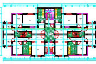
REZ DE CHAUSSEE
