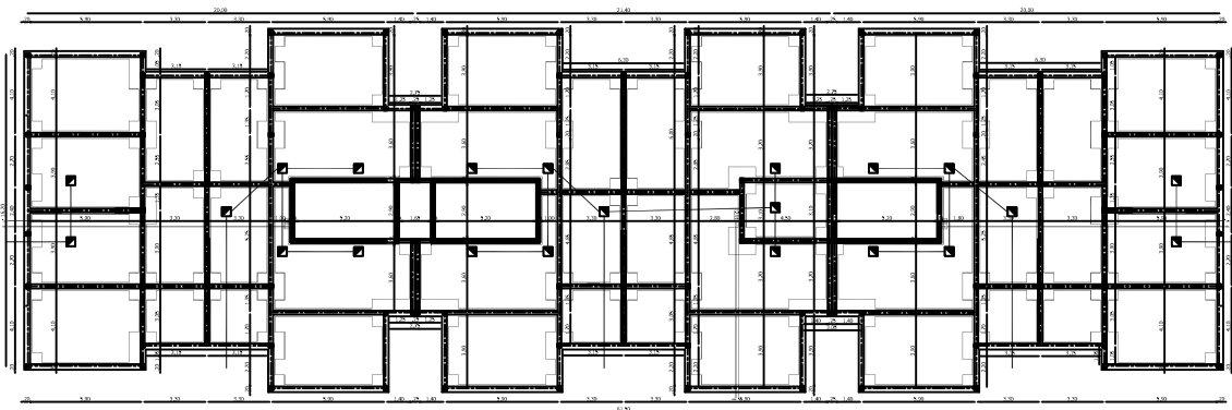
FONDATIONS
