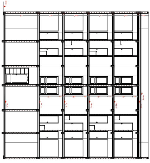
Coupes A/A
