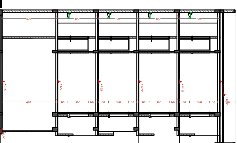
Coupe A-A
