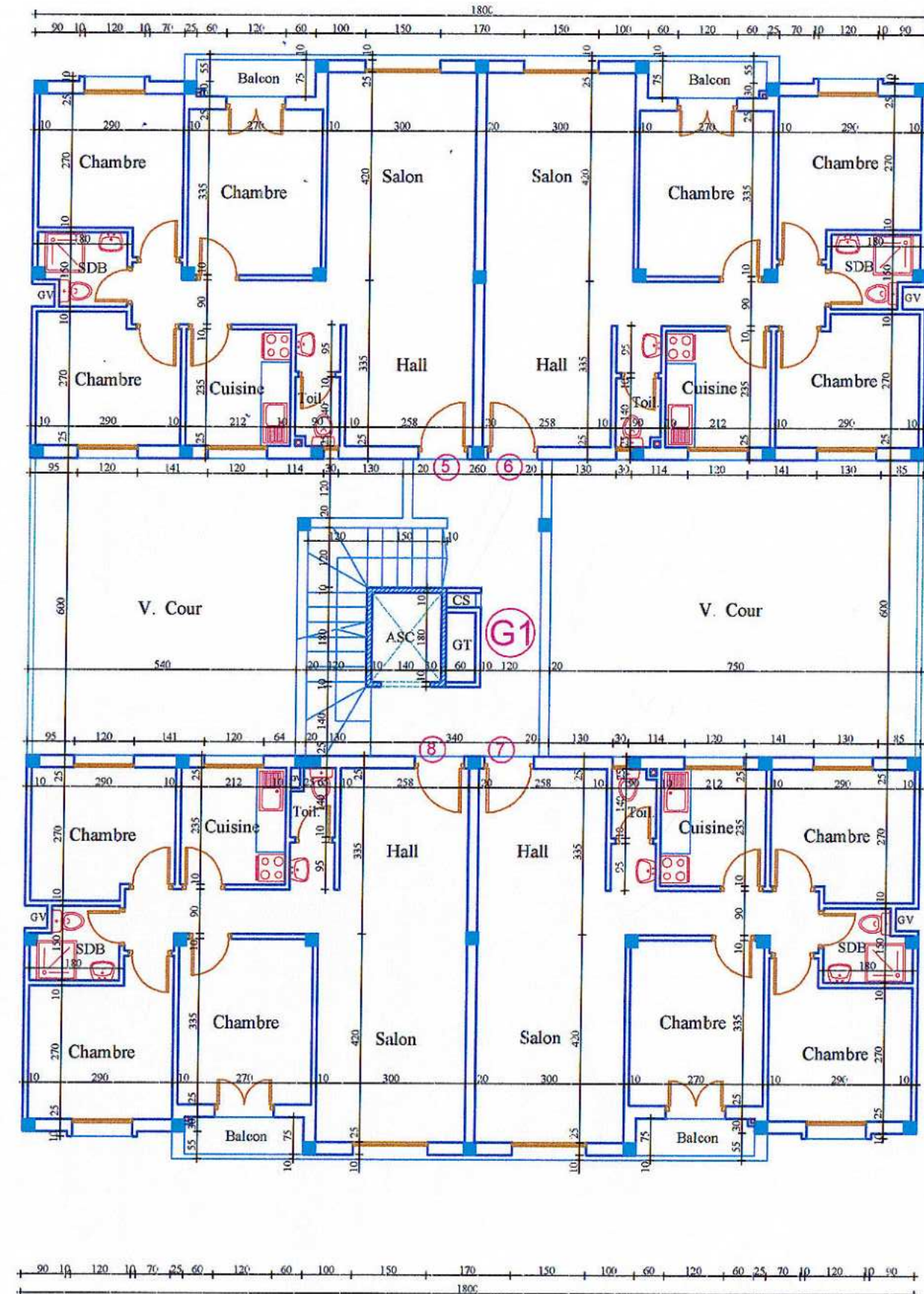
1er ETAGE - IMMEUBLE G -
