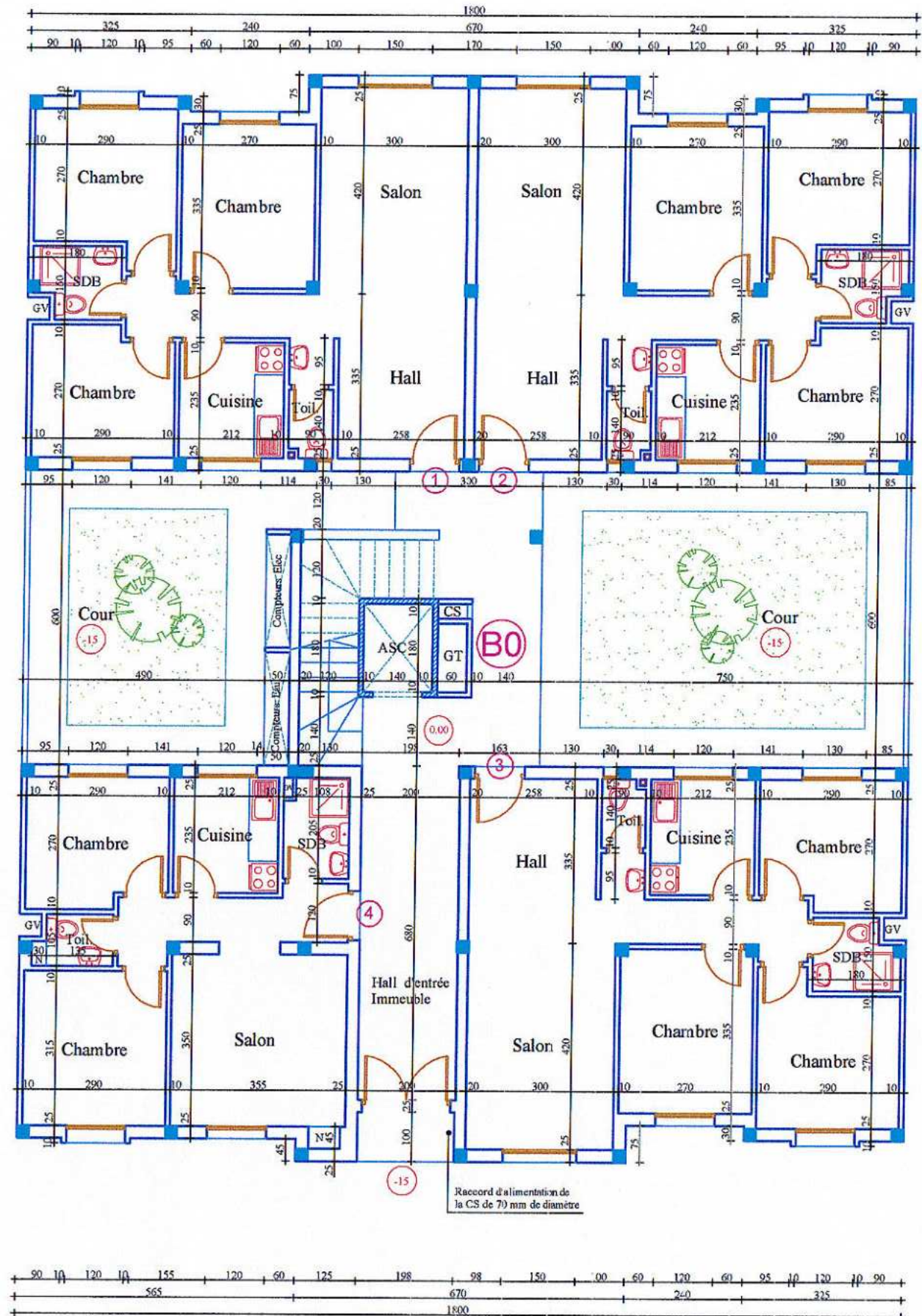
REZ-DE-CHAUSSEE - IMMEUBLE B -
