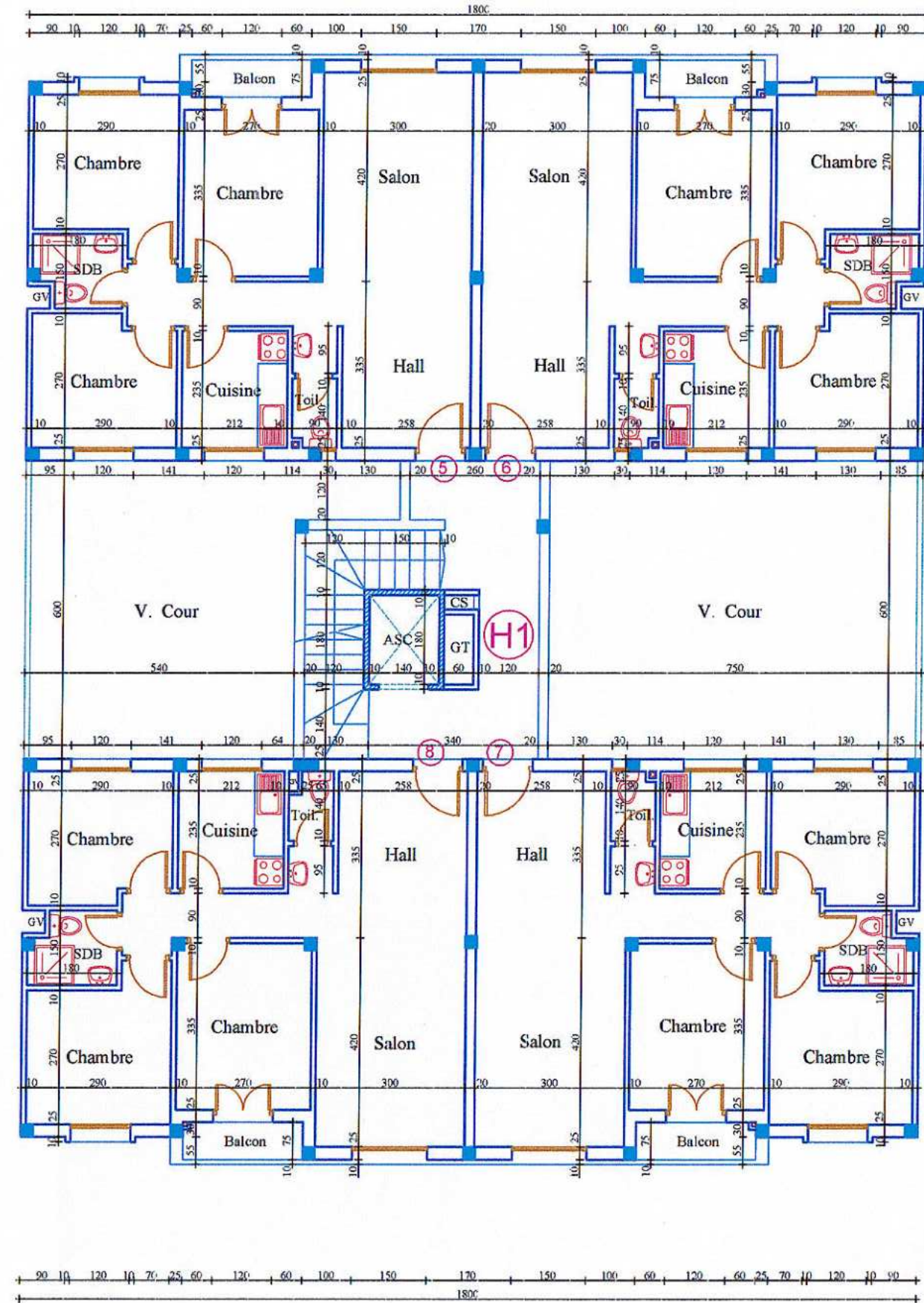
1er ETAGE - IMMEUBLE H -
