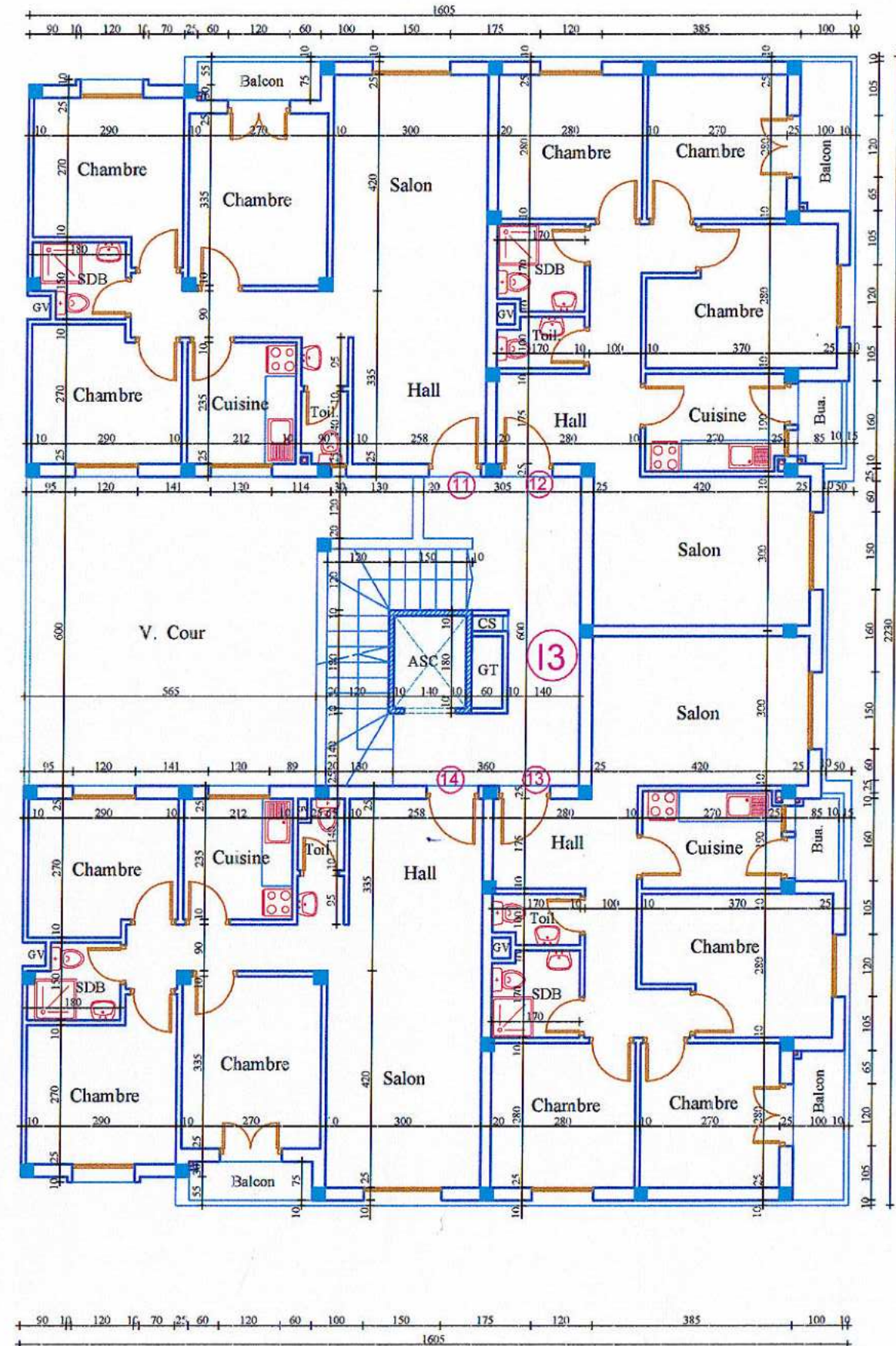
3ème ETAGE - IMMEUBLE I -
