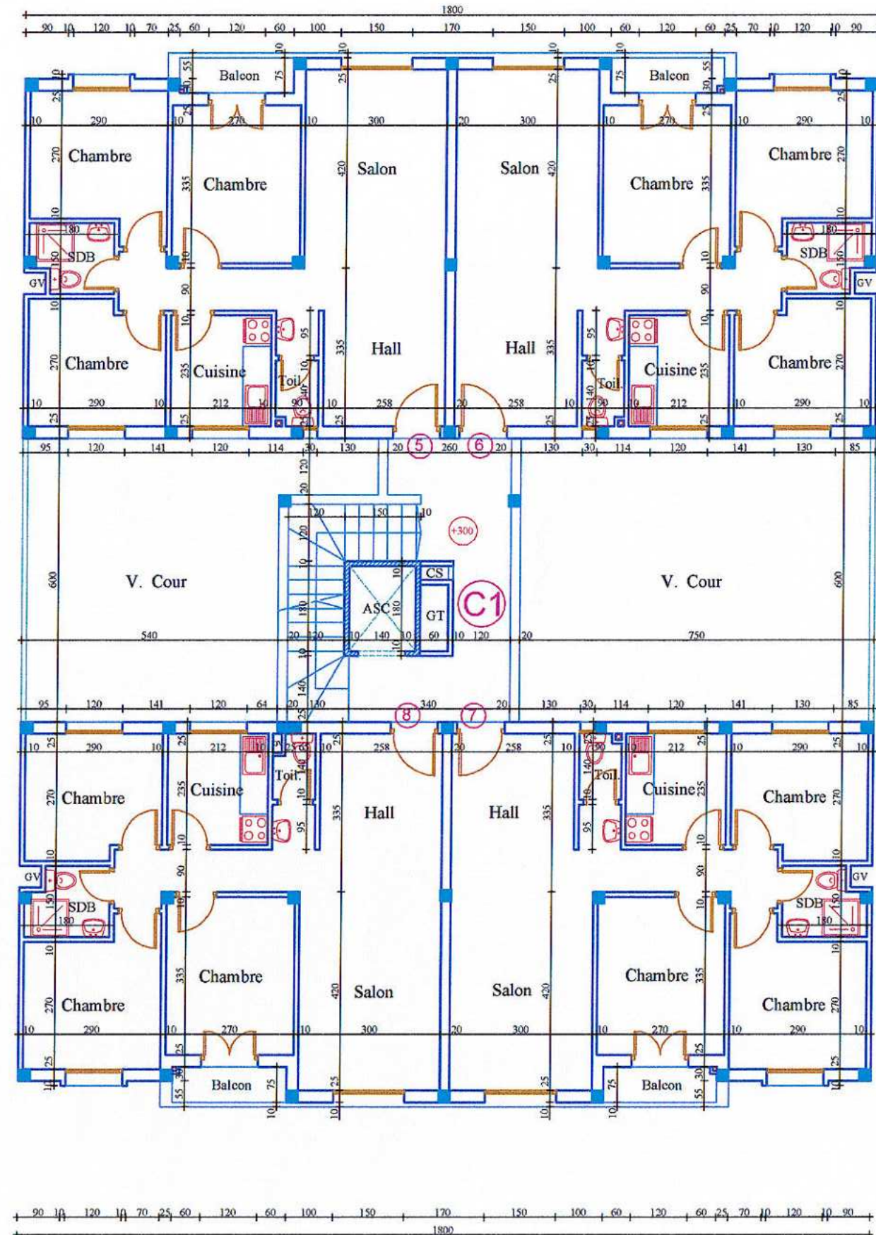
1er ETAGE - IMMEUBLE C -
