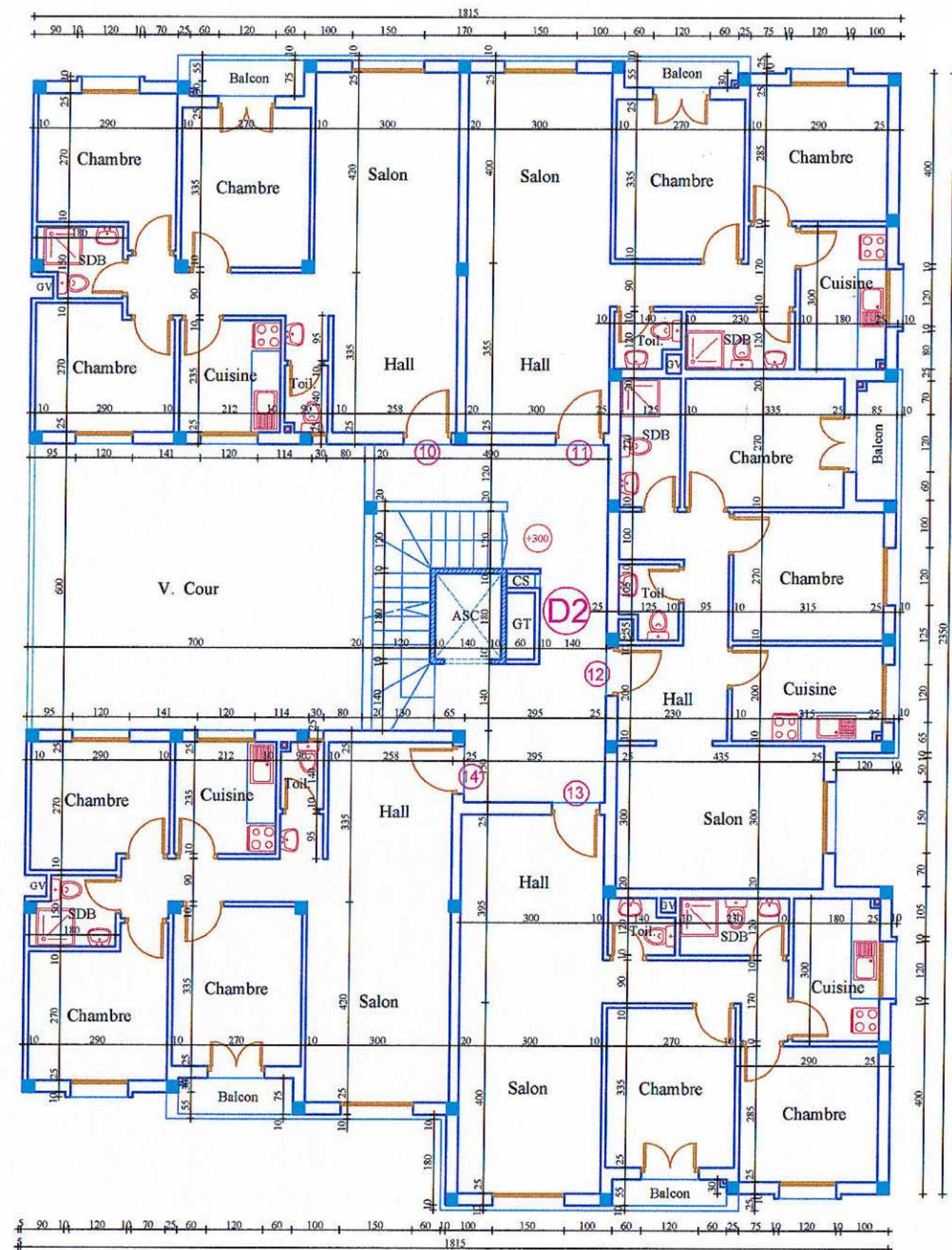
2ème ETAGE - IMMEUBLE D -
