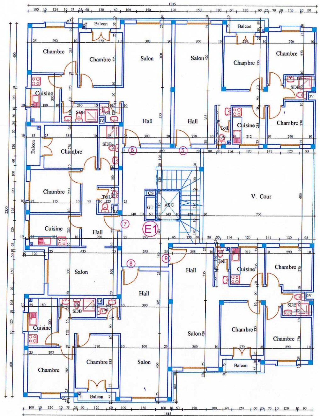
1er ETAGE - IMMEUBLE E -
