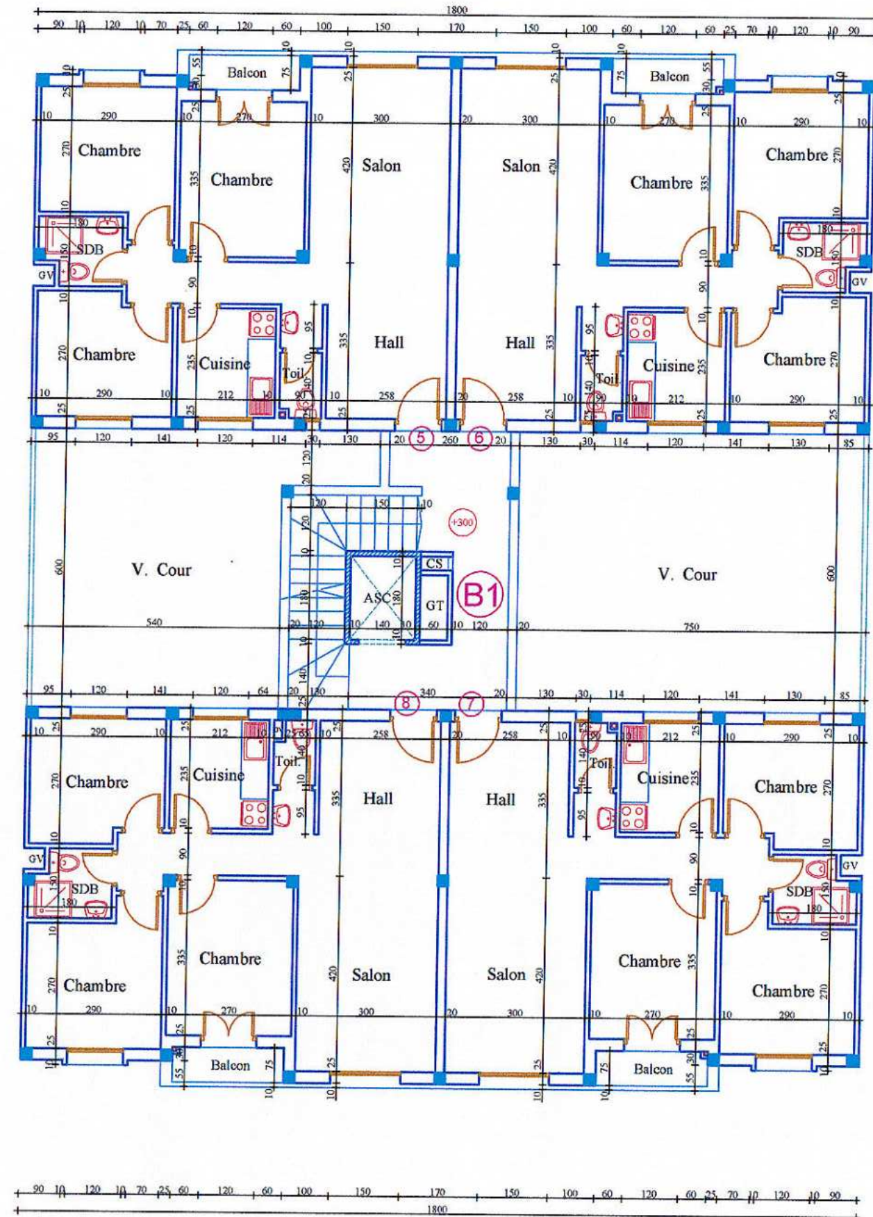
1er ETAGE - IMMEUBLE B -
