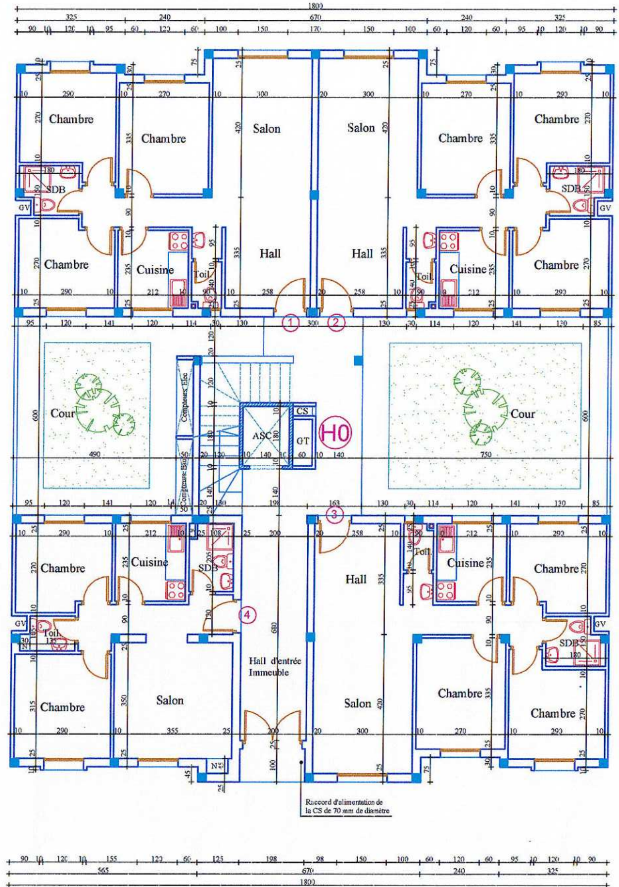
REZ-DE-CHAUSSEE - IMMEUBLE H -
