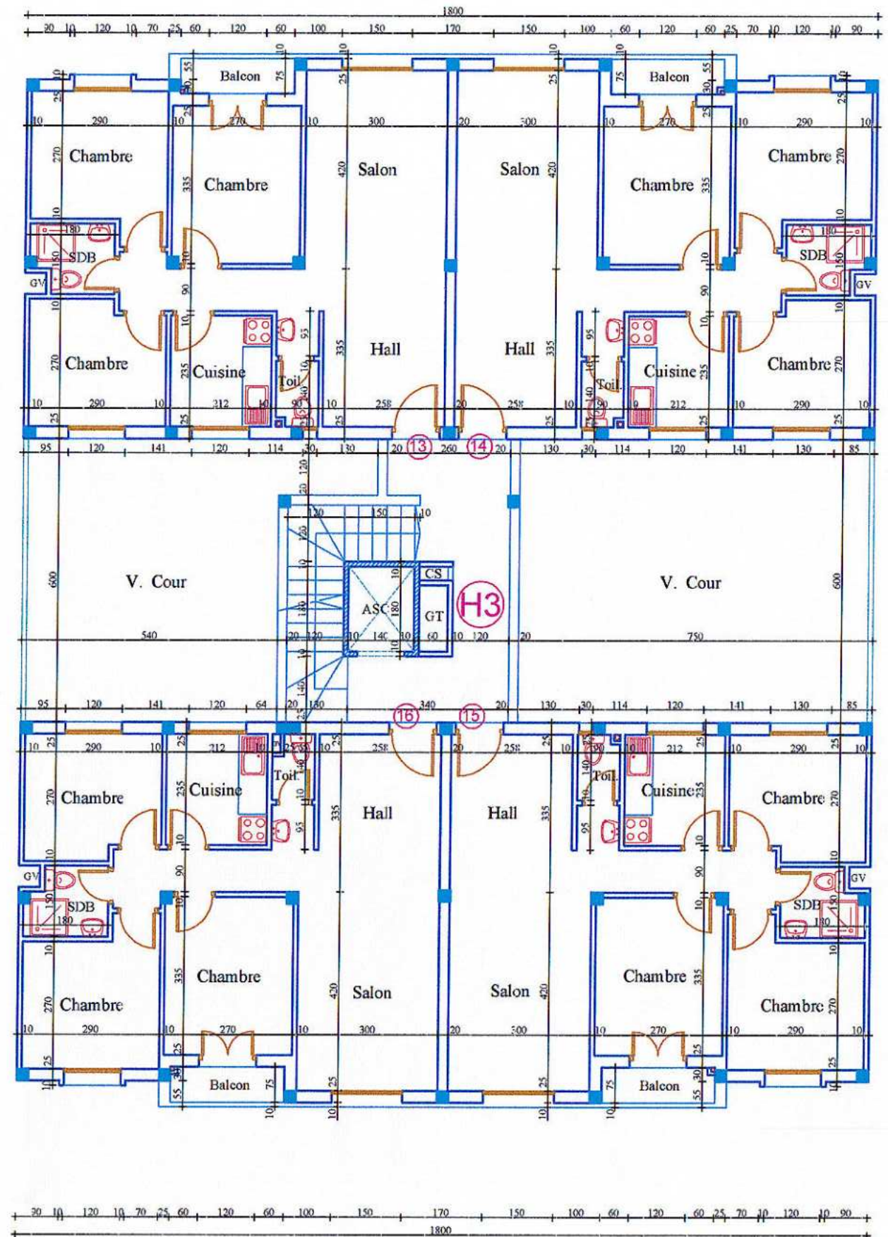
3ème ÉTAGE - IMMEUBLE H -
