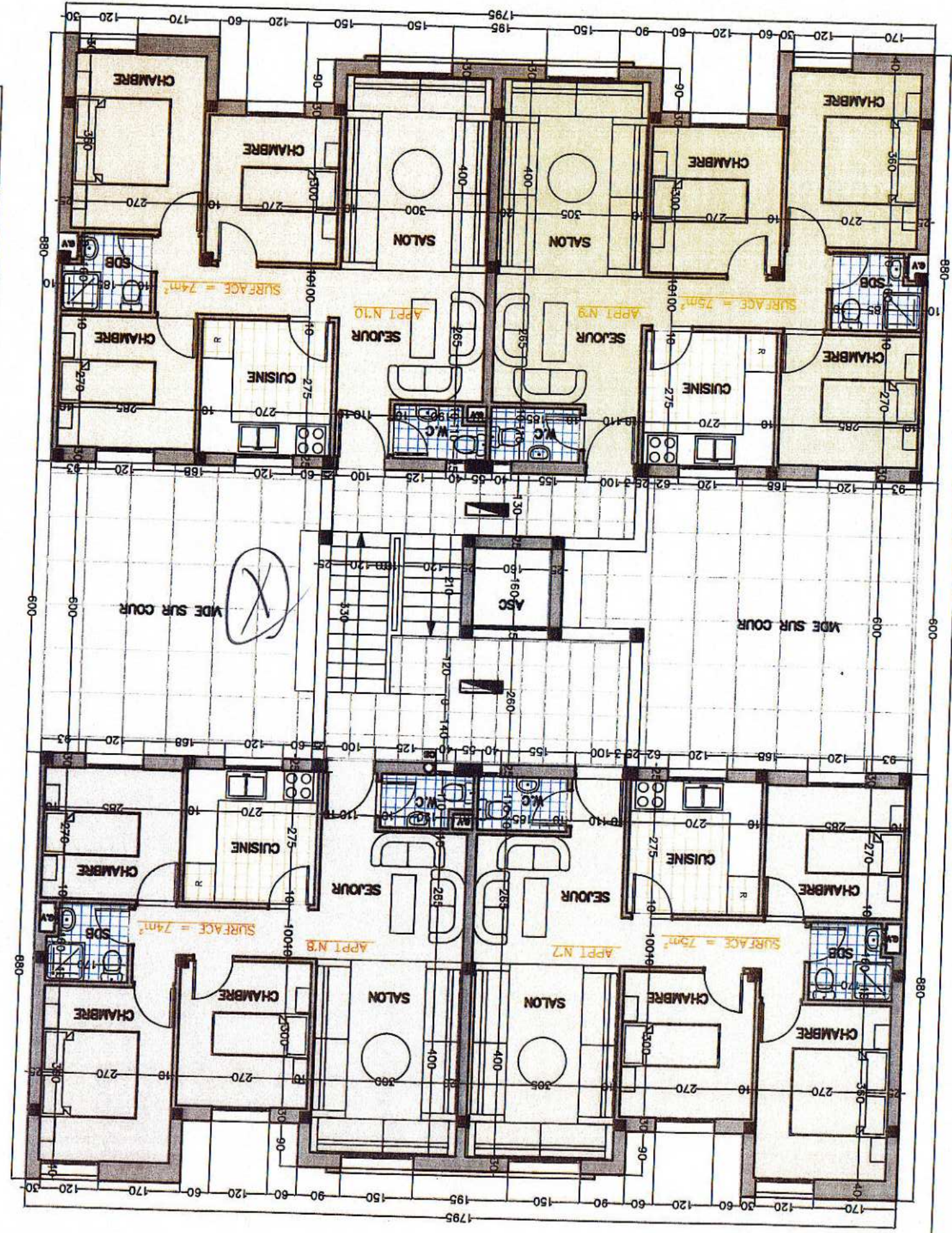
PLAN 2ième ETAGE BLOC E
